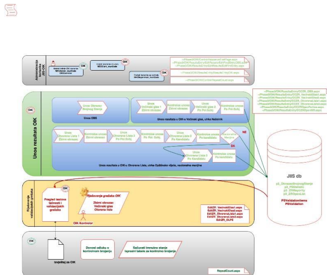
Слика7. Дијаграм функционалних цјелина новог модула
