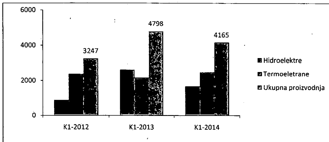
Grafikon 5: Proizvodnja električne energije u BiH u GWH
